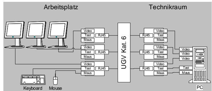
Prinzipaufbau
