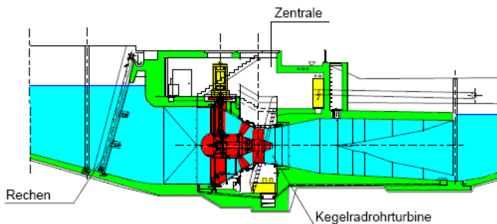
Längsschnitt Turbine
